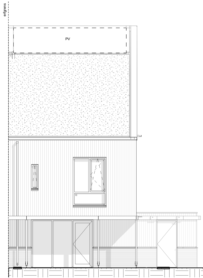
voorgevel (oost)
